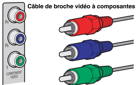
Câble de broche vidéo à composantes
